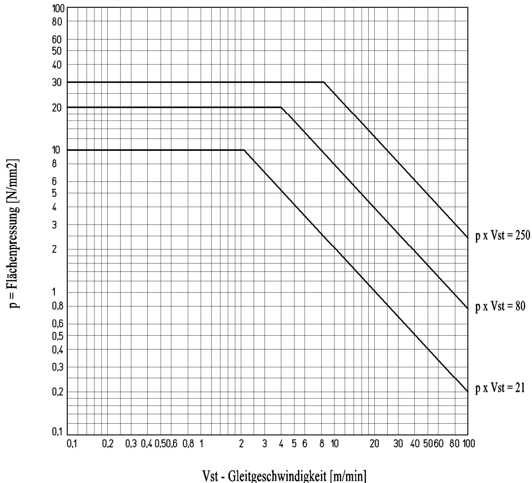
Diagramm Nr. 1 - Gleitbedingungen für Bronze
