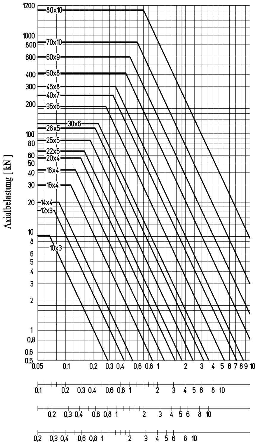
Diagramm Nr. 6 – Spitzenbelastung
