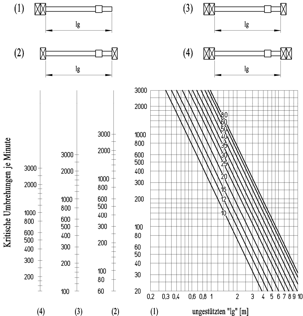
Diagramm Nr. 7 – Kritische Upm
