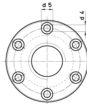
Ab Tr 25x5 (6 bohrungen)
