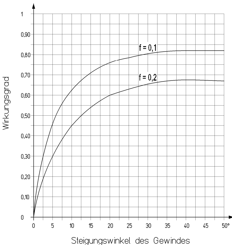
Diagramm Nr. 8: Wirkungsgrad
