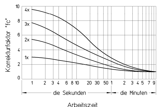
Diagramm n° 5 - Korrekturfaktor " f_c " für Gewindemuttern MPH e FCS
