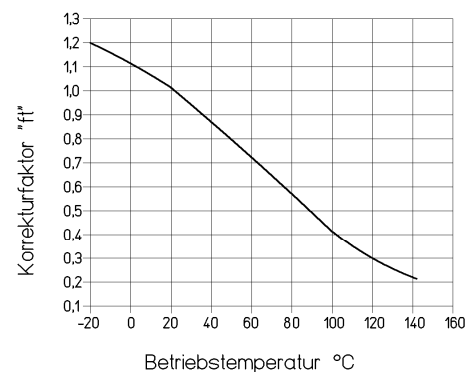
Diagramm n° 4 - Korrekturfaktor " f_t " für Gewindemuttern MPH e FCS
