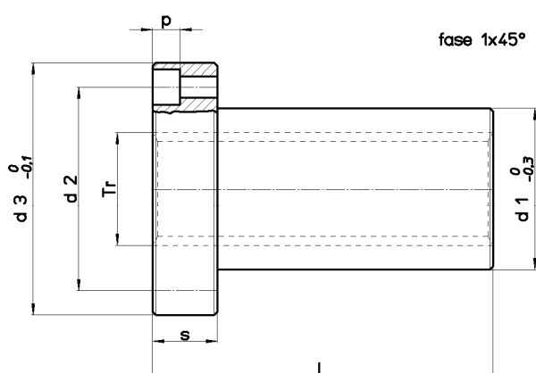
Ab Tr 25x5 (6 bohrungen)
