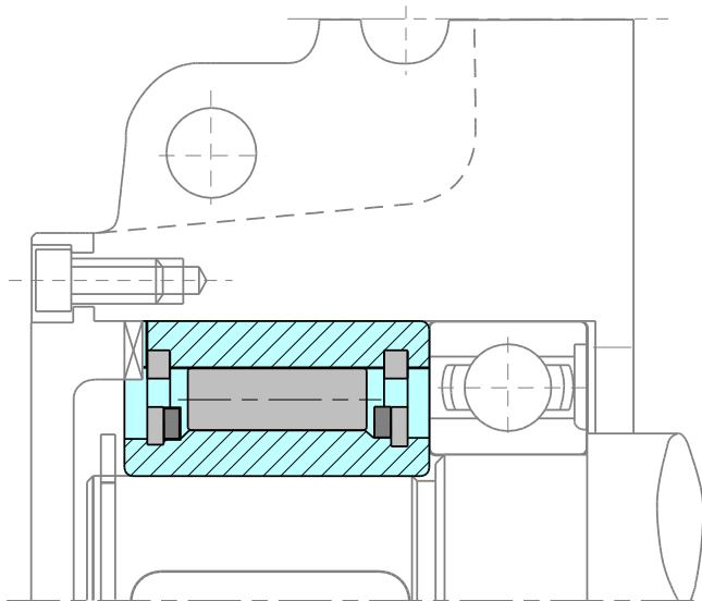
Abb. 3: Einbaubeispiel ASNU
